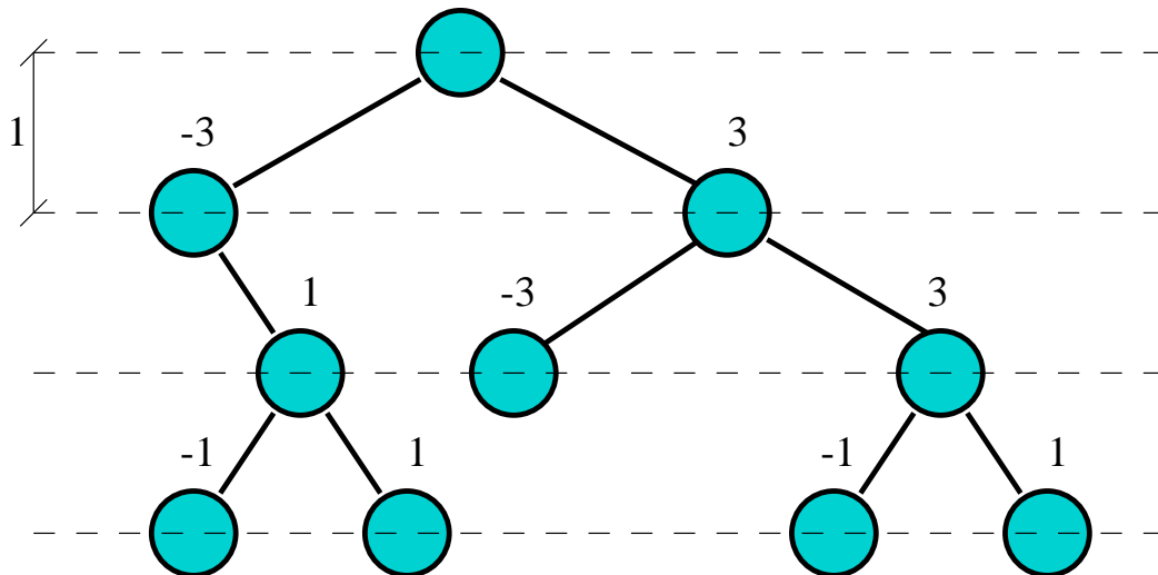
Abbildung 1: Beispiel für ein hierarchisches Layout eines Baumes
