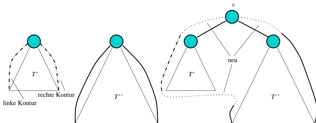
Abbildung 2: Zwei Teilbäume zusammenfügen
